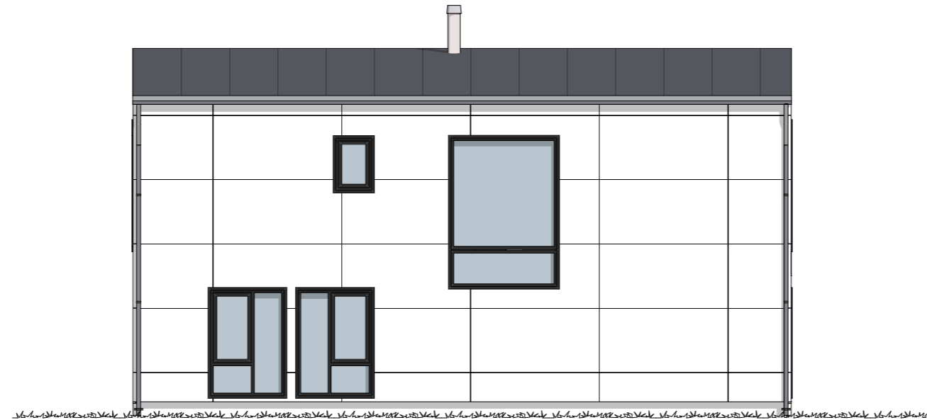
1:100 Fasade 1
